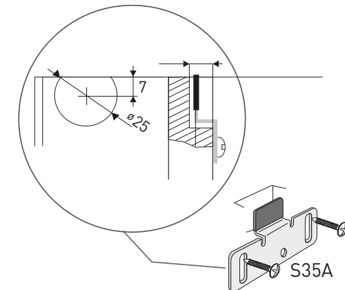
Zafrézování pro horní vozík S35A
