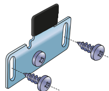
horní vozík S35B bez zafrézování
