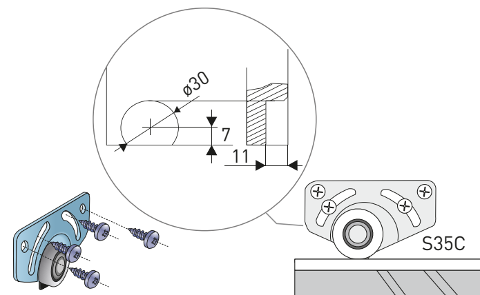
Zafrézování pro dolní vozík
