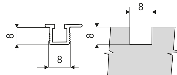
Šířka a hloubka zafrézování pro vodící profil
