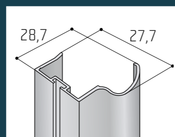
profil S13B
