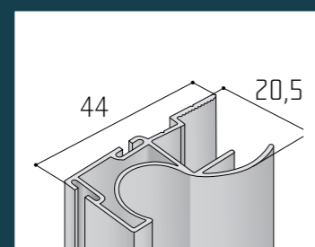
profil S12
