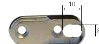
Držák LED šatní tyče a šatního oválu 17D1SWSZ030
