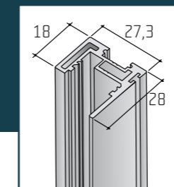
madlo S45B
