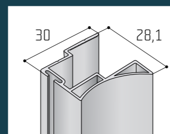
profil S14
