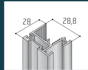
profil S10N
