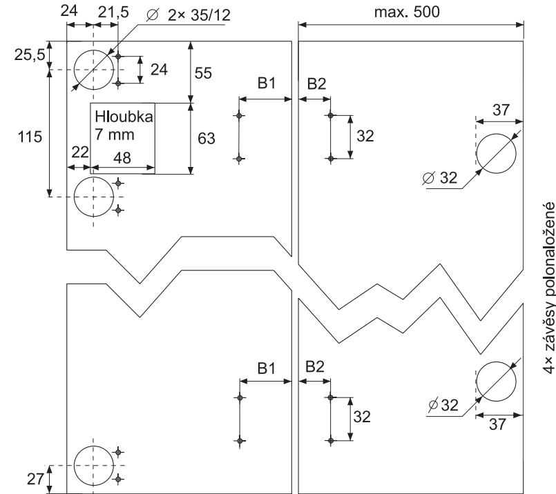
VRTACÍ PLÁN POHLED ZE ZADU
