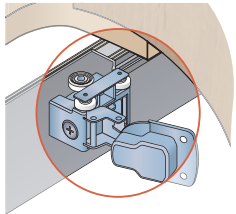
Detail dolního vozíku
